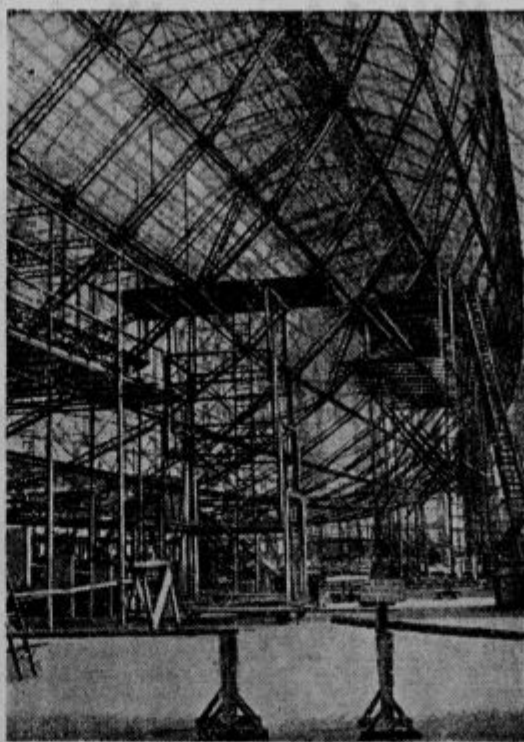
Ogrodje za novi zeppelin »L. Z. 129«, ki bo večji nego vsi njegovi predhodniki. — Ogrodje je iz aluminija.
