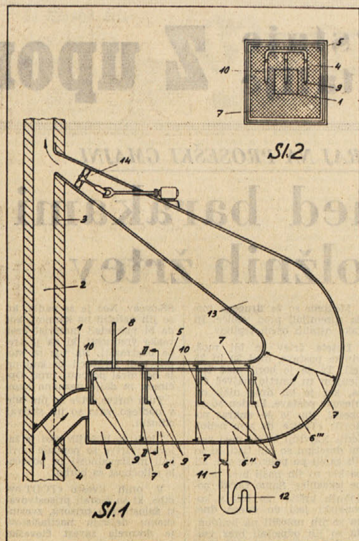
Načrt naprave za «precejanje» saj
