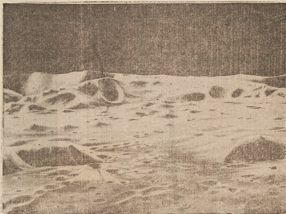
KRAJ PRISTANKA APOLLO 16 NA LUNI — Slika kaže lunsko pokrajino, kjer je pristalo lunsko vozilo Apollo 16. Na levi zadaj je North Ray krater s Smokey gorami (na levi spredaj) proti severu, v sredini kraj pristanka, na desni pa South Ray krater in Stony gore (spredaj).
