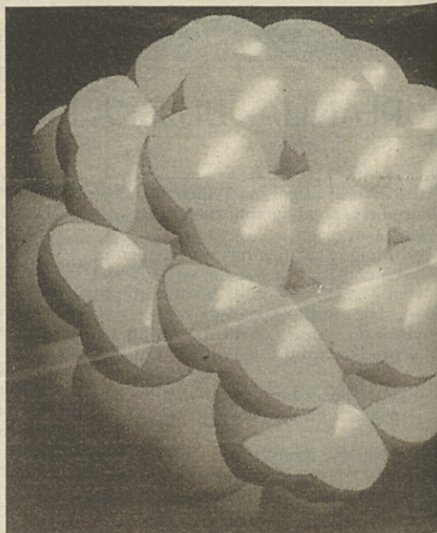
Računalniška simulacija snovi, ki je trša od diamanta.
