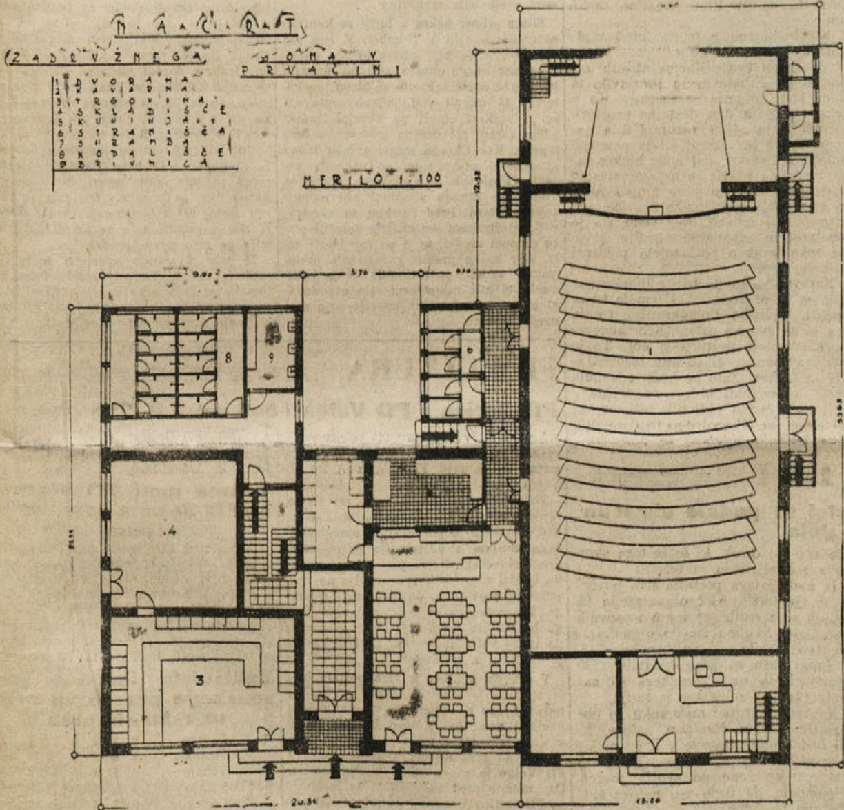
Floris pritičja zadružnega doma Edvarda Kardelja v Prvačini. V domu bodo v pritičju poleg velike dvorane tudi zadružna trgovina, kavarna in kopališče.
