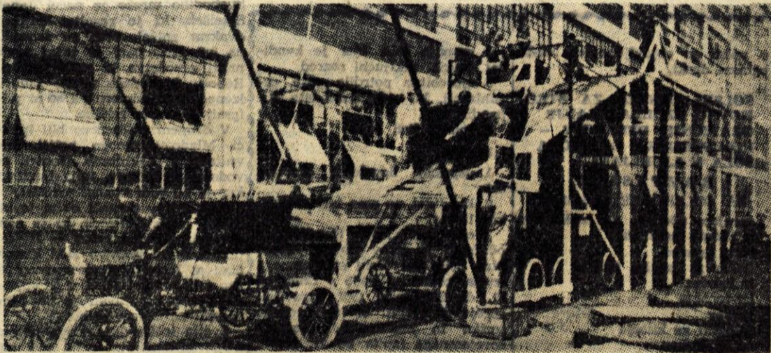
V letih 1914 in 1915 je Ford razširil delo na tekočem traku najprej od zaganjačev na sasilje, potem pa še na montiranje karoserij na sasilje. V sedmih mesecih so skrajšali čas montaže enega avtomobila od 12 ur na 25 minut! Slike, ki kažejo takratne proizvodne postopke, nam danes sicer izvajajo nasmeji: začetek pa je bil le storjen, neprekinjena proizvodnja na tekočem traku
