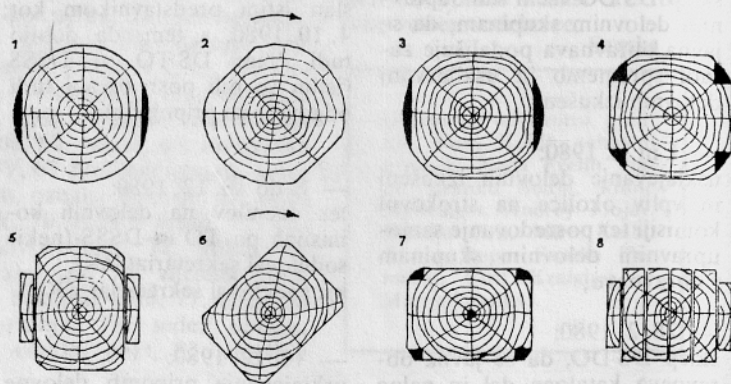
Princip obdelave oblovine s profilno tehnologijo
