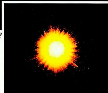
Zakaj je v vesolju več materije kot antimaterije?
