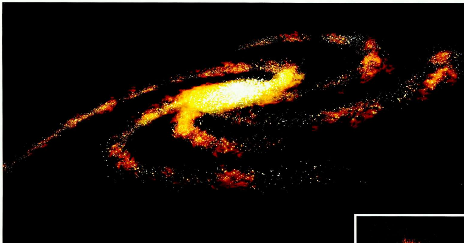
Zakaj je v vesolju več materije kot antimaterije?
