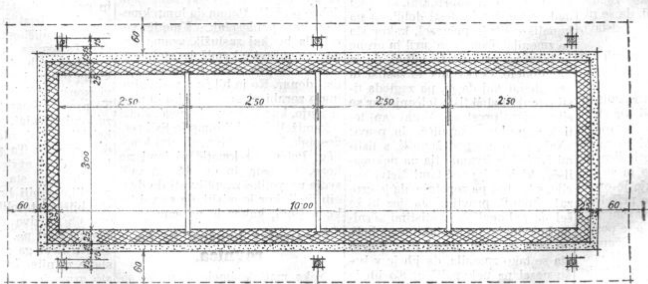
Grundriß
