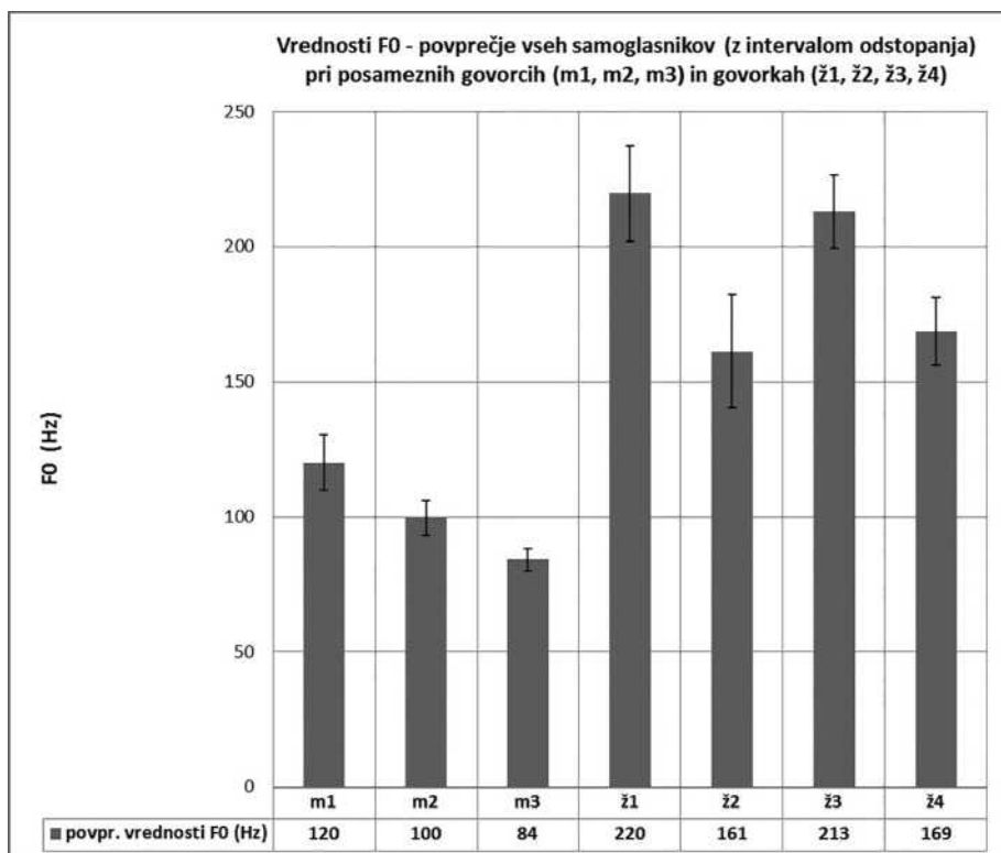
Graf 1: Vrednosti F_0 , izračunane kot povprečje meritev F_0 za vse samoglasnike pri govoricah in govorkah, analiziranih v okviru doktorske disertacije (Tivadar 2008).
