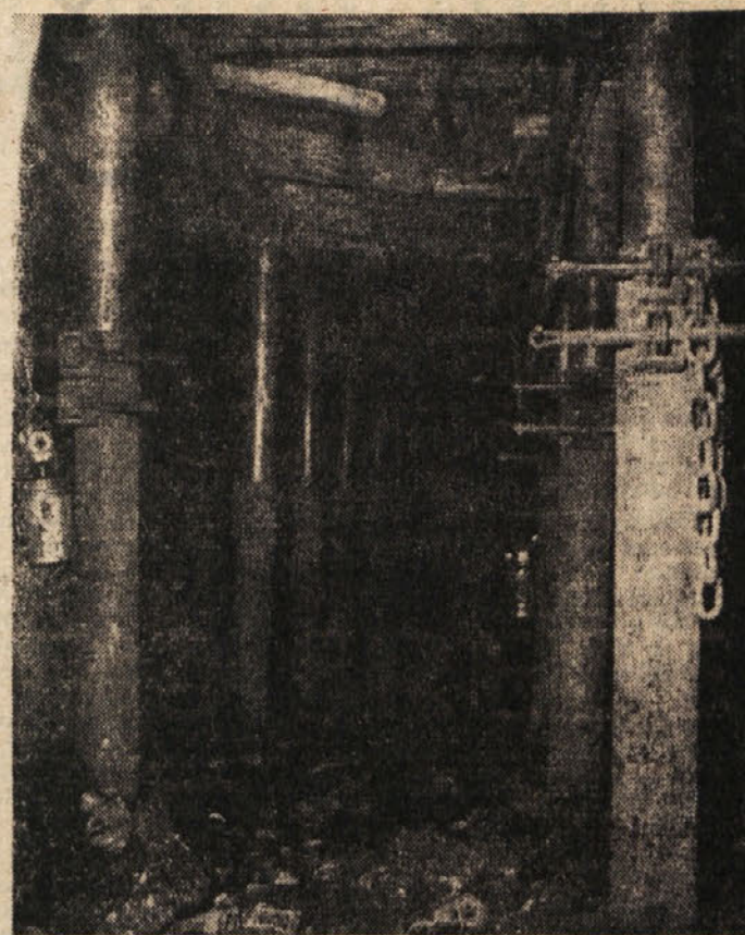
ZELEZNE JAMSKÉ STOLKE — IZDELEK STT, KI SE VEDNO BOLJ UVELJAVLJAJO
