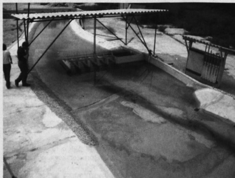
Raziskovalci s pomočjo hipermangana, ki vodo obarva, opazujejo, kolikšen del vodnega toka gre v obtočni kanal, kolikšen pa skozi prelivna polja.
