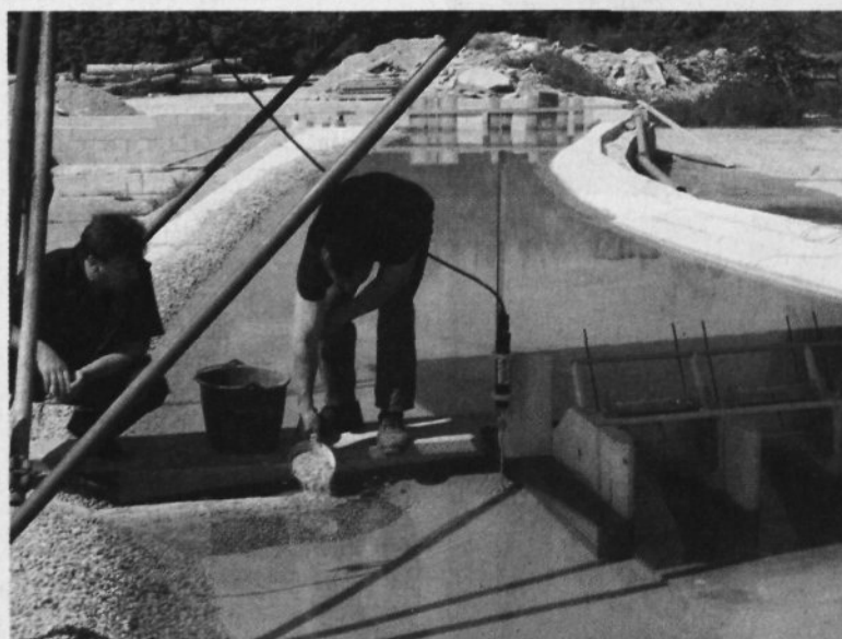
Tako na modelu HE Blanca raziskovalci »gradijo« nasip za preusmeritev vodnega toka na strojnični objekt. En jogurtov lonček materiala pomeni en tovrstjak materiala v naravi.
