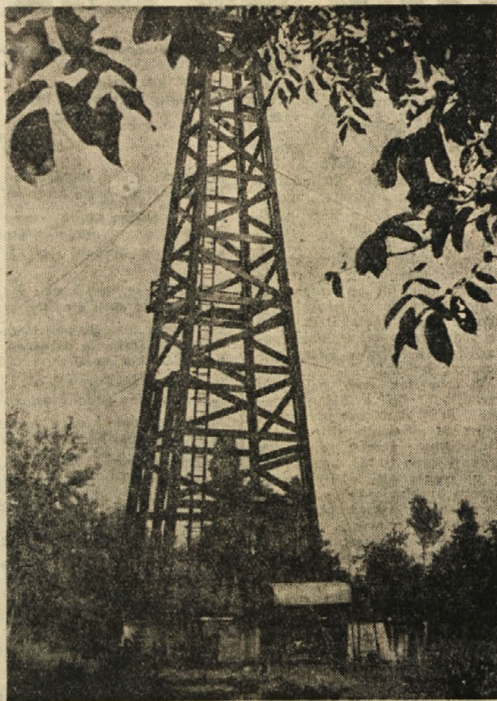
Ekspluatacijski stoip v Lendavi z globinsko črpalko
