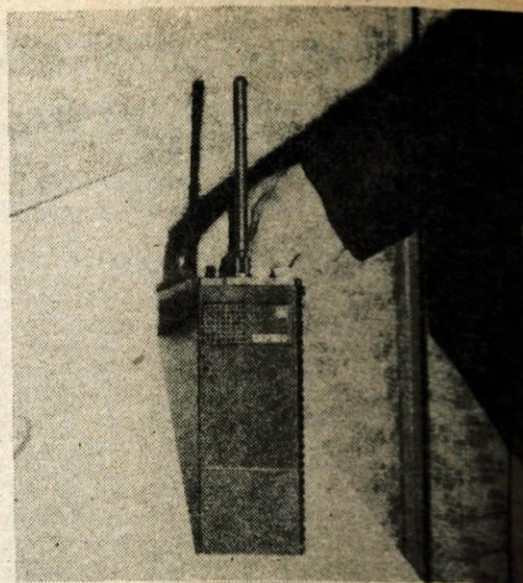
Ročna sprejemno-oddajna postaja tipa UKP 700 predstavlja novo generacijo prenosnih postaj. S svojimi izvedenkami UKP 720, UKP 740 in UKP 760 pokriva celotno frekvenčno področje, namenjeno mobilnim radijskim zvezam. Aparatura je namenjena za brezžični govorni promet med prenosnimi, mobilnimi ali fiksnimi postajami.
