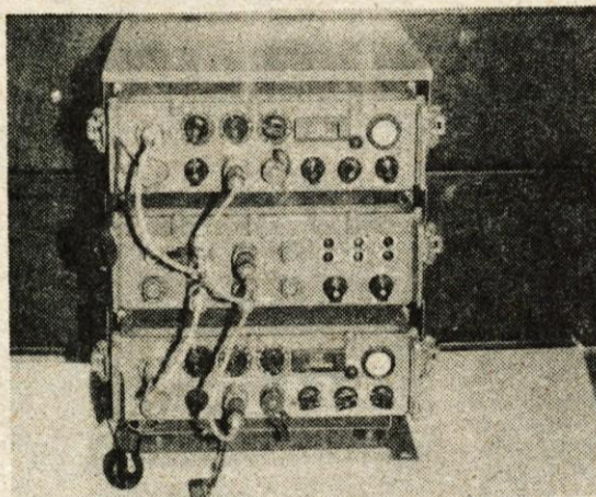
Sistem Sora za avtomatsko retranslacijo z eno anteno v frekvenčnem področju 34-37 MHz je namenjen razširitvi radio mreže, ki se zaradi velikih razdalj ali naravnih preprek ne more direktno povezati. Omogočeno je hkratno delo na dveh sistemih RUP-20 na isti anteni. Sistem SORA povezuje radio-mreže, ki delajo z različnimi vrstami modulacije.
