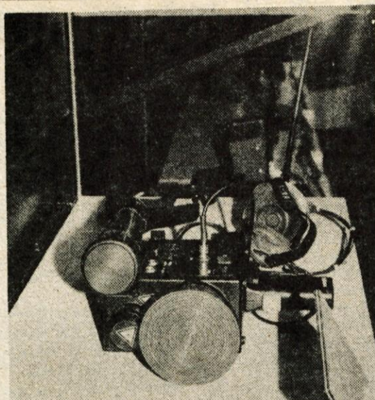
Laserski komunikator je namenjen vzpostavljanju telekomunikacijskih zvez za srednje in kratke razdalje. Njegovim zvezam je nemogoče prisluškovati. Ima prenosno in fiksno izvedbo. Zveze se vzpostavljajo hitro in enostavno.
