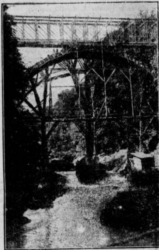
Betoniranje oboka mostu.
