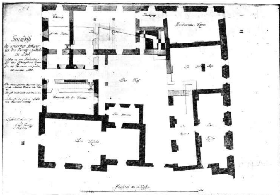
Ptoris pritličja starih in novih špitalskih poslopjij po načrtu iz 1791. (Original v Arhivu Slovenije v Ljubljani.)
