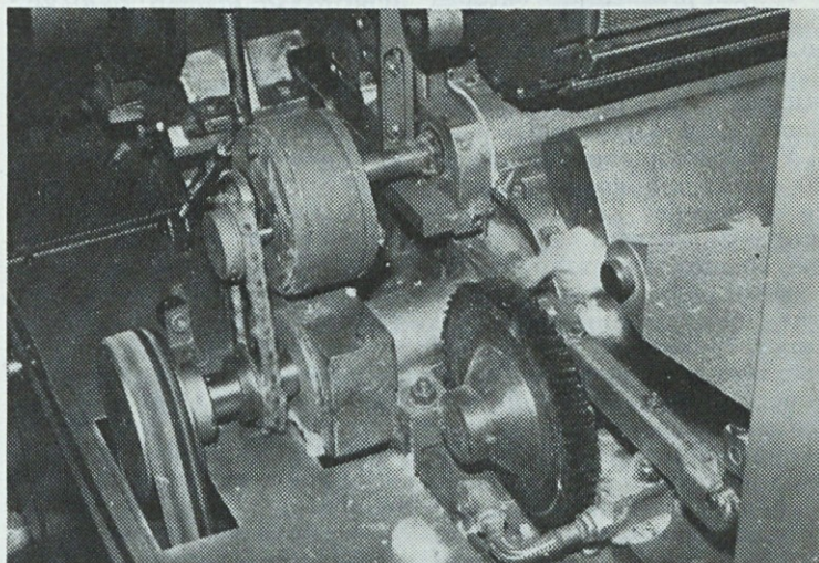
Na 8. mikalniku Platt smo, ob snemalnem valju, namestili foto celico, ki ob debelejši plasti nabranih vlaken, avtomatsko izključi mikalnik in tako prepreči uničenje garniture. Na posameznih mestih mikalnika je izpopolnjeno izpraševanje in dovajanje bombažnih vlaken v mikalnik. V kopreni mikalnika je manj nopkov (smeti). Dosežena je večja enakomernost mikalnikovega pramena.
