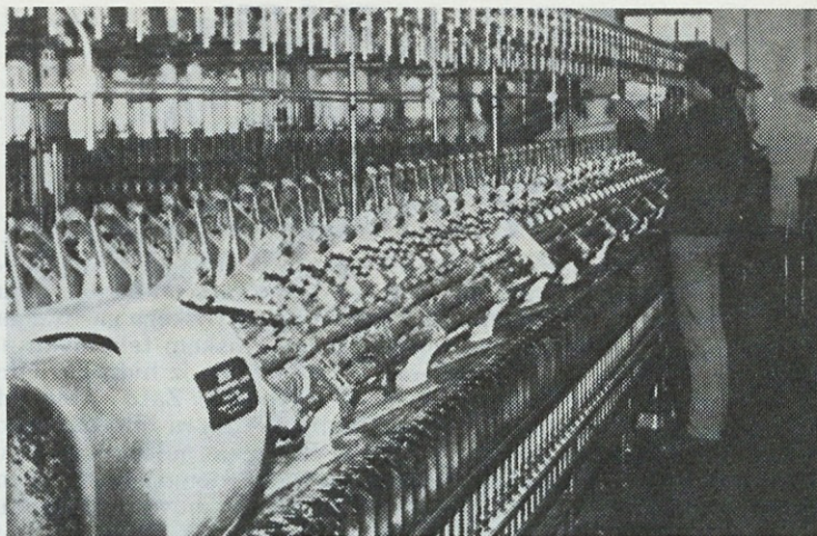
Demontirani prstančni stroj Ingolstadt smo začasno montirali v predilnici IV. Prizadevamo si, da ob zamenjavi prstančnih strojev proizvodnja preje ne bo manjša.
