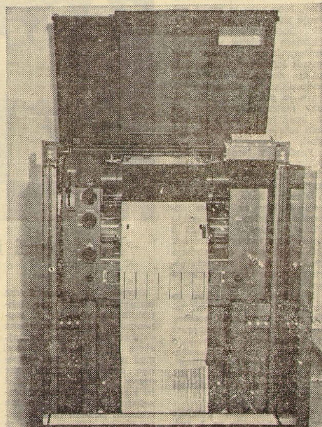
Zgornji posnetek predstavlja hitri pisalnik v centru za avtomatsko obdelavo podatkov. Njegova zmogljivost je neverjetno velika — tisoč vrstic v eni minuti
