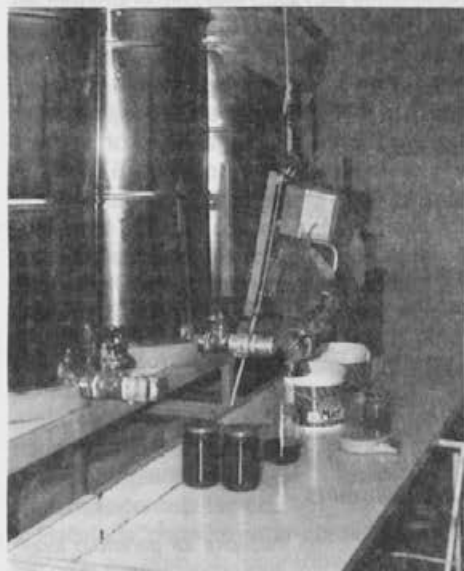
Enostavna naprava za doziranje medu, ki se montira direktno na zorilne posode ali kar na sode. Zelo je praktična in natančna.
