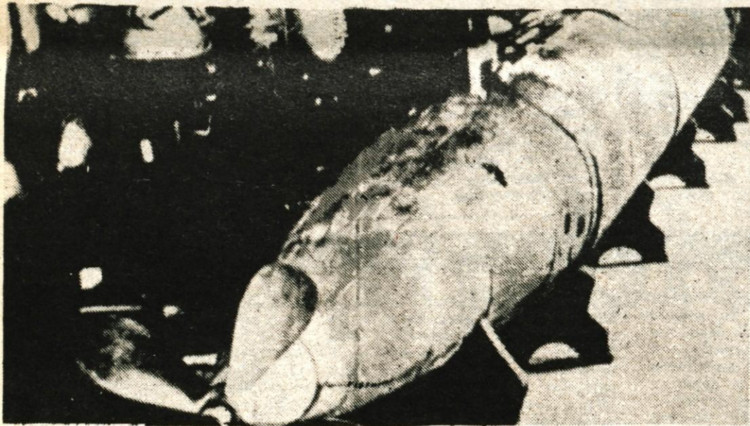
Mina, kakršno so Italijani uporabili v napadu na Viribus unitis v puljskem pristanišču.
