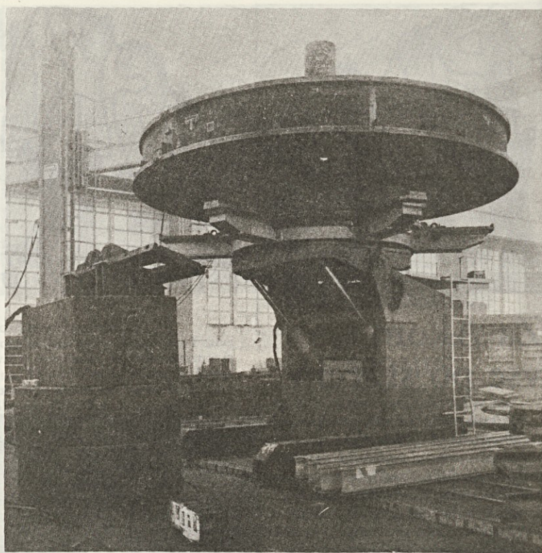
Turbinski pokrov, montiran na pozicionerju POH 500, je pripravljen za nadaljnjo obdelavo
