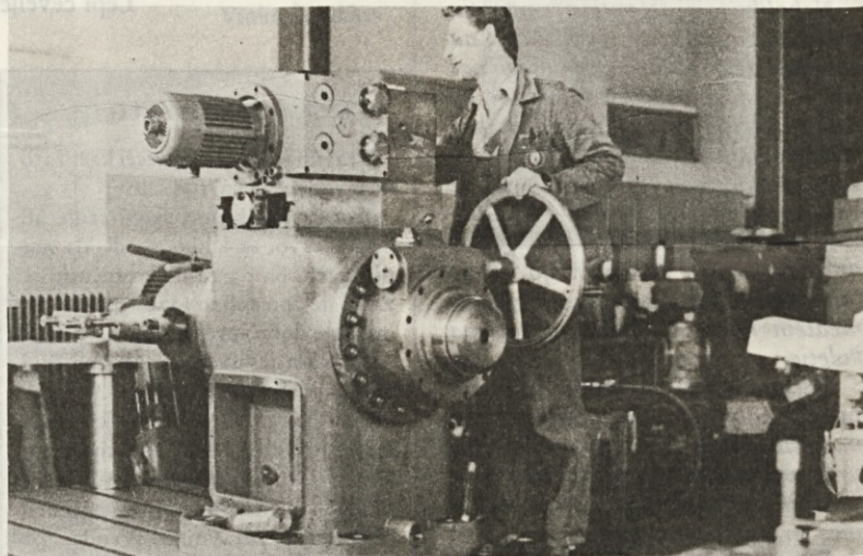
Avtomatski regulator vrtilne hitrosti za HE Tis Abbay — Etiopia za tretjo Francisovo turbino moči 3956 kW. Standardni regulator za 250 — 3000 3000 kgm s krmilnim regulatorjem AT-5 v sestavi pred funkcijskim preizkusom. Prva dva agregata uspešno obratujeta v Etiopiji že 20 let. Investitor je naročil še tretji agregat. Zdaj končujemo delo na zadnji opremi, v drugi polovici tega leta pa bomo montirali opremo v Etiopiji in vstavili v obratovanje še tretji agregat.
