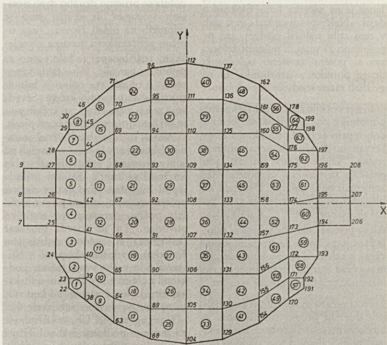
Razdelitev plošče zapiralnega telesa na elemente
