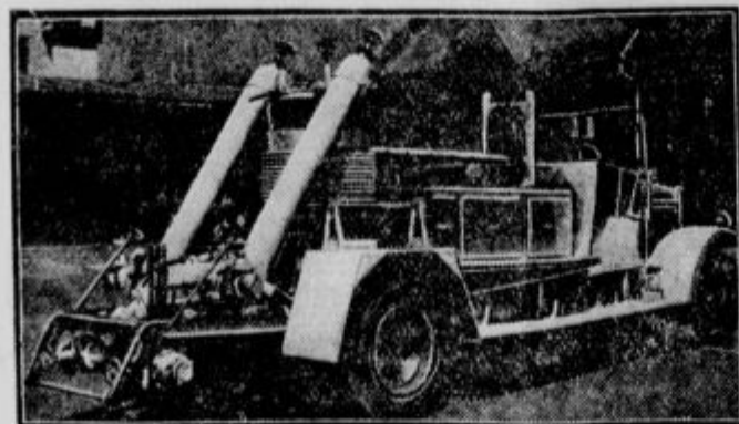
Brizgalna za gašenje ognja s prahom. Brizgalno bodo uporabljali tam, kjer bi voda napravila veliko škodo: v trgovinah za manufakture, papirjem itd.. Gasilna mešanica sestoji iz ogljikove kisline in natrona.
