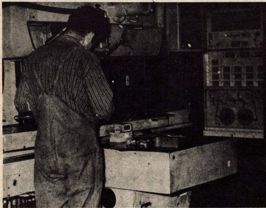
Med najsodobnejšo strojno opremo ima IKOS tudi 2 numerično krmiljena rezkalna stroja, ki po pripravljenem programu lahko s šestimi upetimi orodji opravita tudi po deset in več zahtevnih operacij brez posredovanja delavca. Uporablja jih za izdelovanje najzahtevnejših strojnih delov, ki terjajo največjo možno natančnost. Foto: S. Hain
