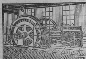
LANZ'sche Heißdampf-Ventil-Lokomobilen mit direkt gekuppelter Dynamo.
