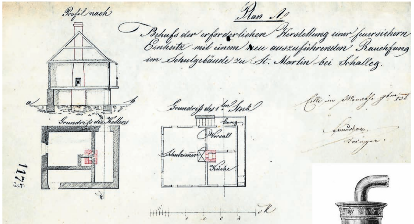
Načrt ureditve dimnika šolskega poslopja – Sv. Martin pri Šaleku. Vir: SI_ZAC/0008, Okrožni urad Celje
