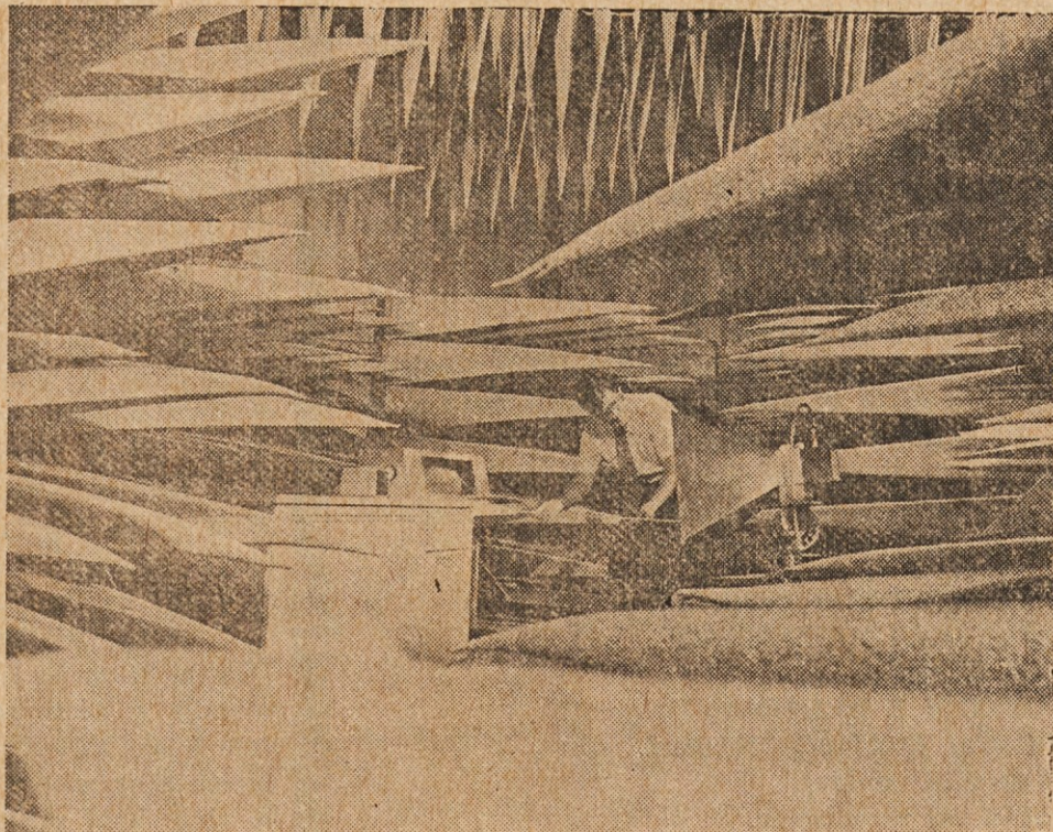
PRESKUSEVALISČE — Prostor s 6 čevljev v dolgimi ostrimi stožci je urejen za preskušanje računalnikov IBM v Rochesteru, N.Y. Ti stožci zmanjšujejo odbijanje elektronskih signalov in s tem omogočajo inženirjem preskuse o morebitnih nehotenih signalih, ki jih bi računalniki dajali.
