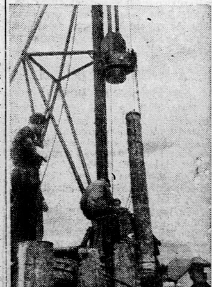
Del stroja za zabijanje pilotov v zemljo
