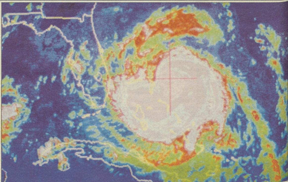
S satelitskega posnetka je zgovorno razvidno, kakšno ogromno razsežnost ima orkan Berta (Telefoto AP)
