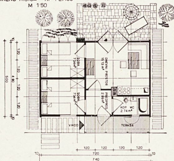
VIKEND HIŠICA TIP PL/100 M 1:50
