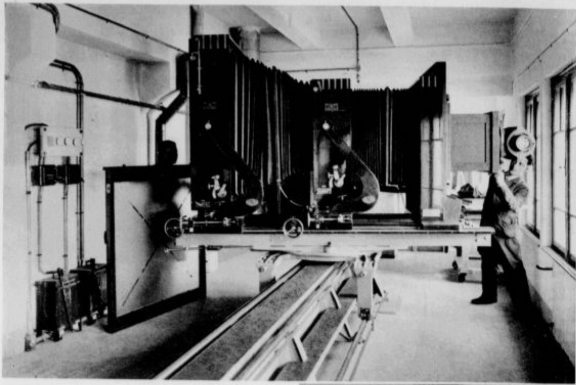
Fotografični aparat, največji in najmodernejši na vzhodu Evrope. Dolžina 8 metrov, klišejska ploskva 120 m x 120 m.
