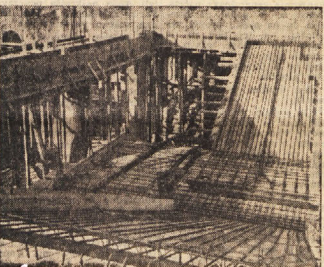
Leseni opaz in položeno železo za stopnišče, ki bo vezalo vhodno halo s halo v prvem nadstropju, iz katere se bo stopalo v parter dvorane.
