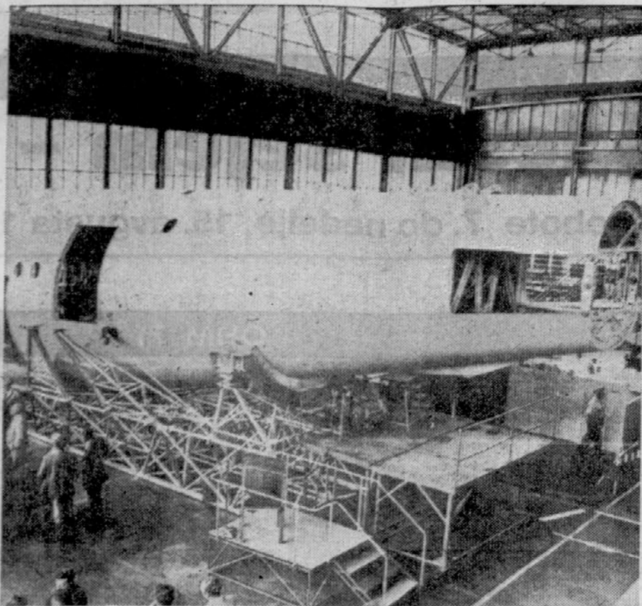
EVROPSKI ZRAČNI AVTOBUS — Ogradje za prototip evropskega zračnega avtobusa s šifro »A 300 B« so pripravili v proizvodni dvorani podjetja Messerschmitt-Bölkow-Blohm v Hamburgu, kjer ga bodo naložili na ladjo in poslali v Bordeaux. Francoska podjetja bodo nadaljevala z gradnjo zračnega velikana. Telefoto: UPI
