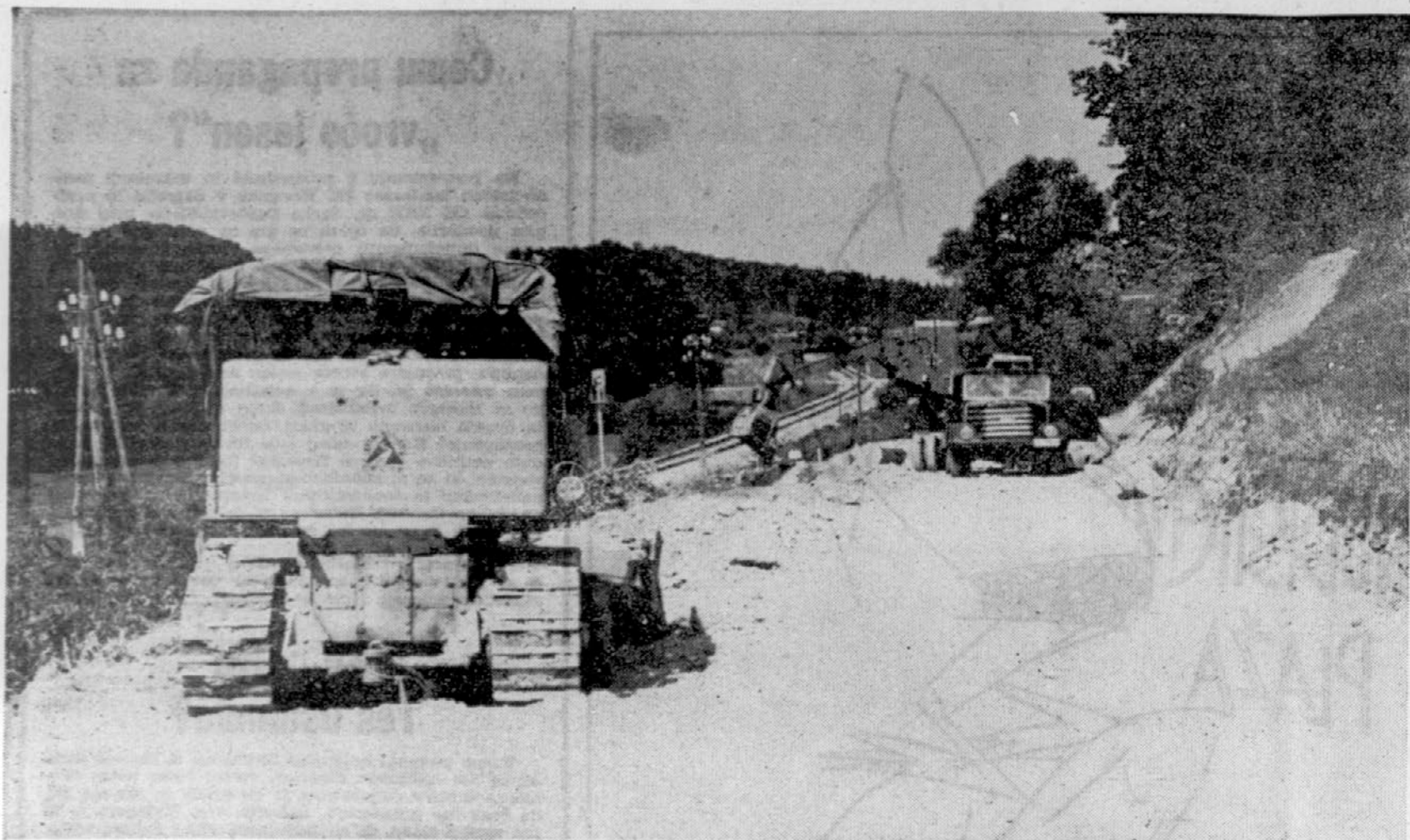
UREJANJE SMEHOVEGA KLANCA — Cestno podjetje iz Celja je začelo urejati Smehov klanec na cesti Celje—Rogaška Slatina. Pri rekonstrukciji 1400 metrov dolgega odseka bo treba nasuti preko 12.000 kubičnih metrov nasipov. Asfaltno prevleko bodo položili do začetka novembra.
