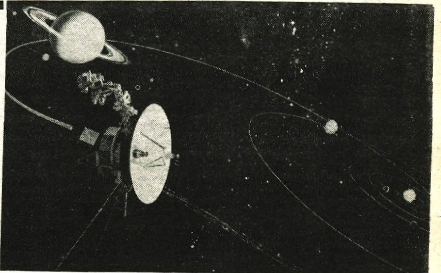
Prikaz poti ameriške sonde Voyager 1, ki je doslej poslala na Zemljo okrog 80 tisoč posnetkov, od tega 20 tisoč s Saturna, s čimer je močno okrepila dosedanje poznavanje tega zanimivega planeta.
