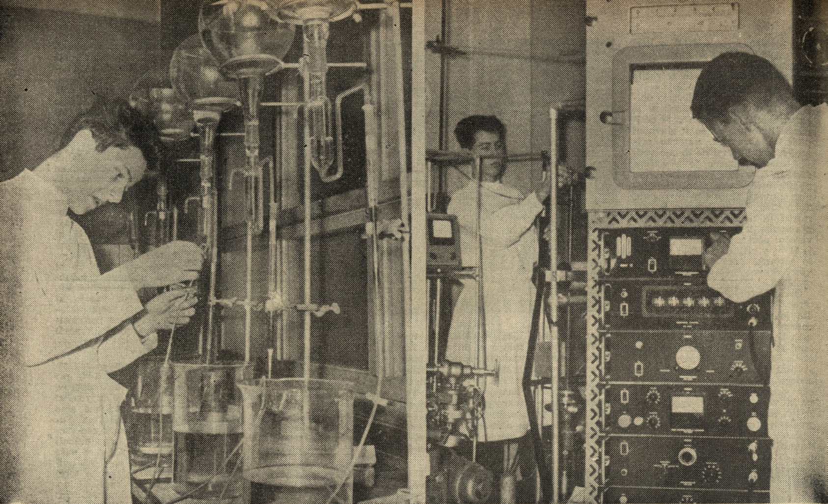
Leva slika nam kaže, kako v švicarskem laboratoriju preizkušajo razne snovi filtrov za odpravljanje radioaktivnosti iz vode po cisternah. Voda teče iz majhnih rezervoarjev skozi filtrirne stolpce v velike steklene posode. — Desno: komplicirana merilna naprava, ki meri razen impulzov tudi moč radioaktivnosti. Tako je mogoče ločevati sevanje različnih radioaktivnih snovi. Tala moderni laboratorij je urejen v Baslu.
