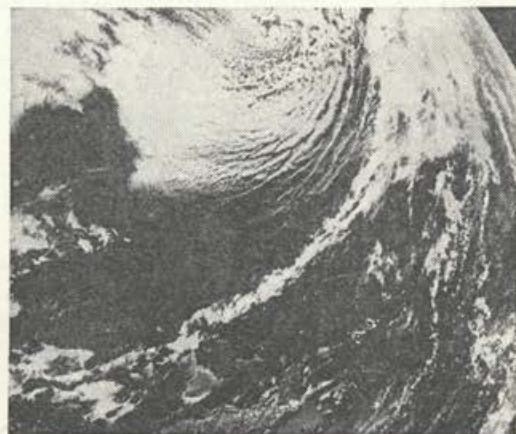
Posnetek Zemlje z višine 1000 km. Jasno se vidijo vrtnčasta oblačna področja, zarodki ciklonskega delovanja
