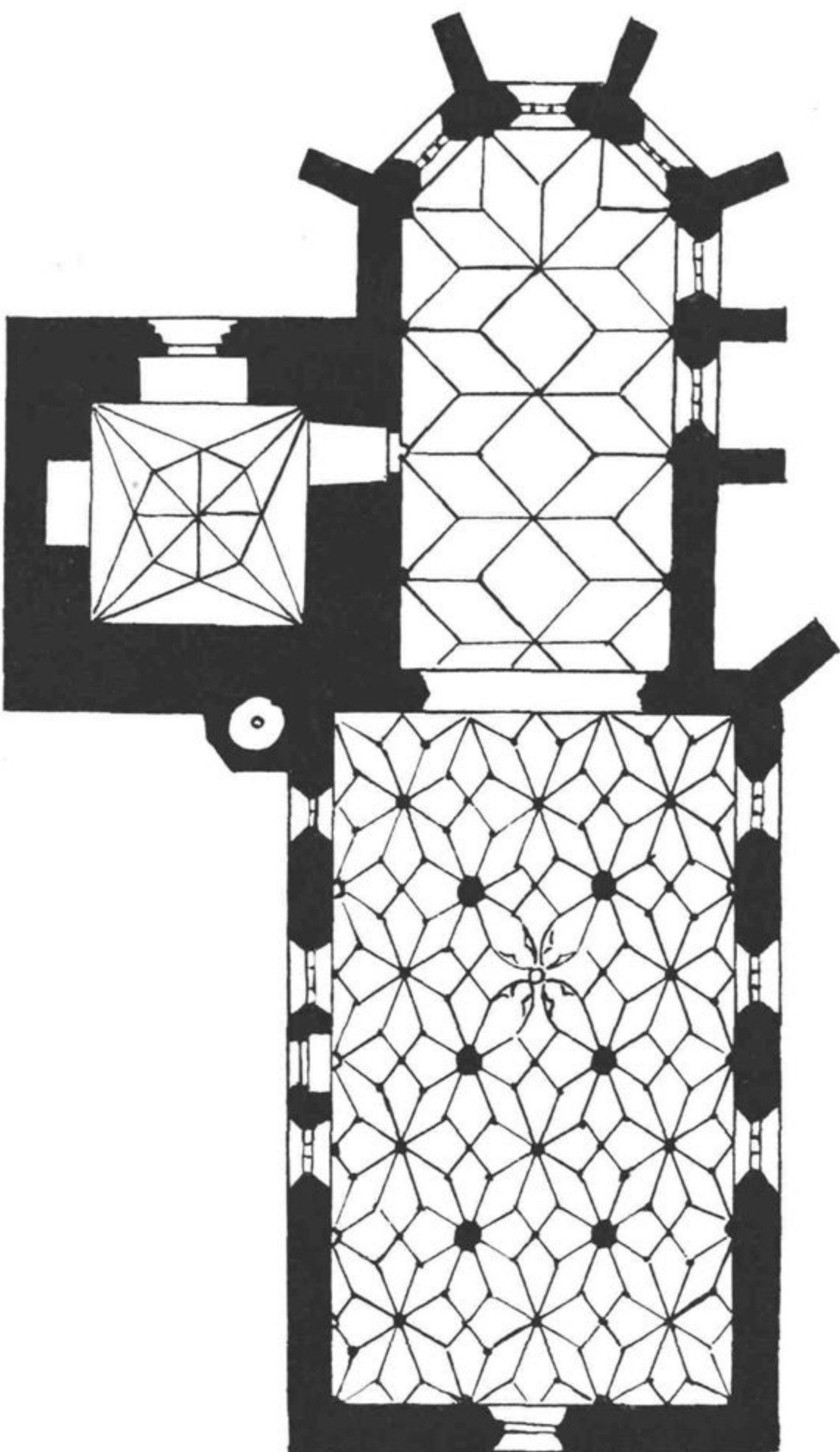
Sl. 1. Šent Rupert: cerkev, talni načrt
