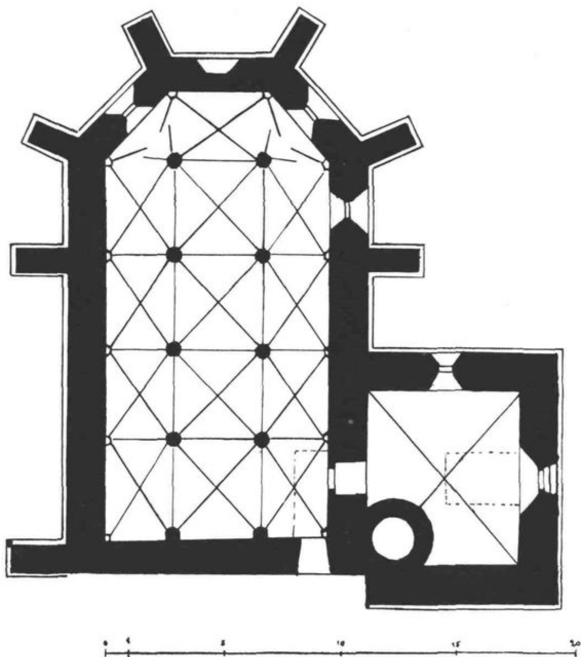
Sl. 4. Kapiteljska cerkev: kripta, talni načrt
