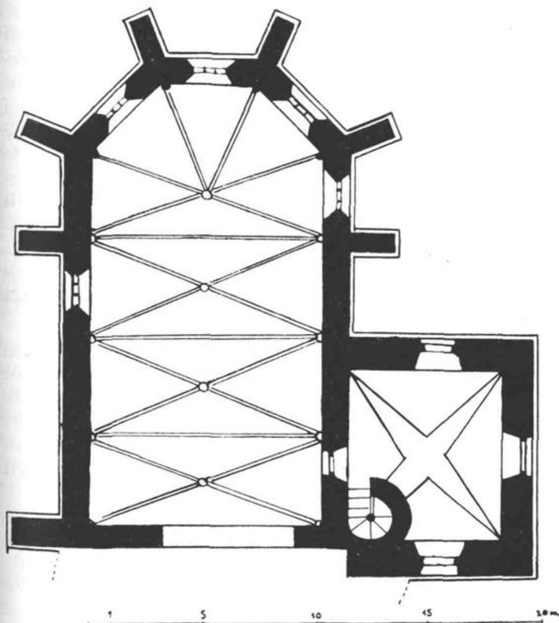
Sl. 2. Kapitljska cerkev: prezbitarij, talni načrt
