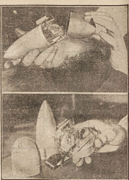
Ija nov aparat za opazovanje vremena, katerega kaže slika. Aparat se nahaja v pločevinasti škatlici. V aparatu je termometer, barometer in higrometer za merjenje vlage. Aparat vzamejo seboj letalci in majhna oddajna aparatura v njem oddaja avtomatično poročilo vsake pol minute o temperaturi, vlagi in zračnem pritisku.
