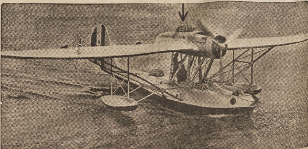
Italijansko letalo Cant Z 501, ki ima Isota-Fraschini motorje s 750 KS, je dosegel nov svetoven rekord. Iz Monfalcone v angleško Somalijo, to je 4966 km, je prevozil v 25 urah. Puščica kaže, kje ima letalo skrito strojnico.
