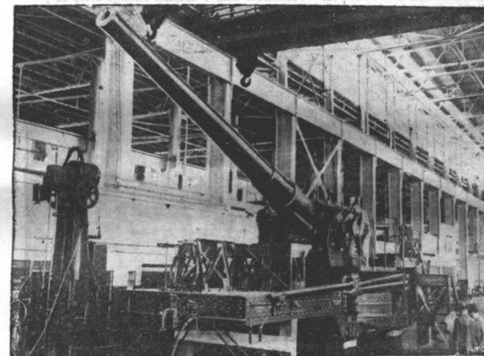
NOV AMERIŠKI TOP. V Waterlownu so zgradili top kalibra 406. Top je montiran na kolesih in odda štiri strele v minuti 50 km daleč
