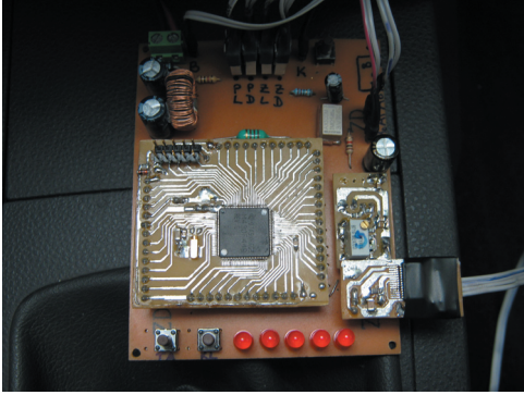
Fig. 4. Controller
