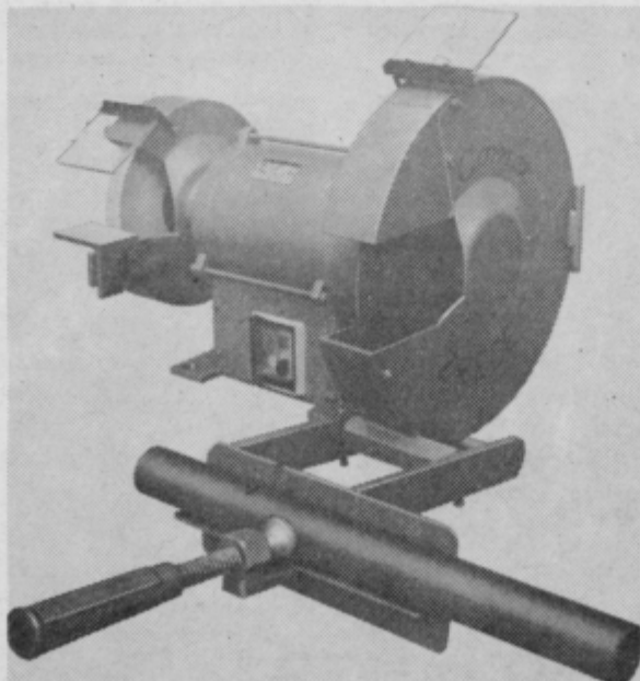
Stroj za brušenje in rezanje BRS 200/300 je novi izdelek proizvodnega programa Cometa, točneje njegovega tozda Conek; pomeni pa tudi izdelek, po katerem vse bolj raste povpraševanje.
