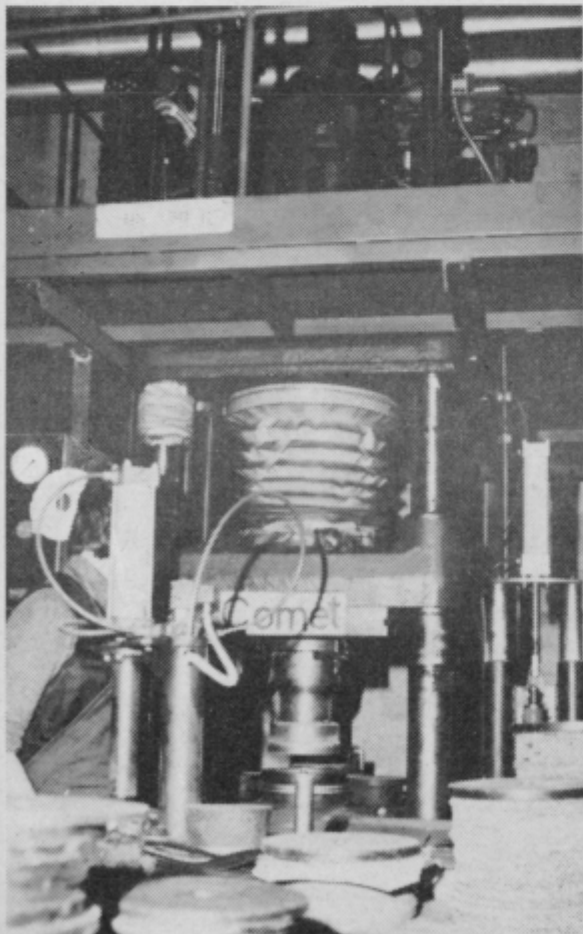
Ob standardnem ogrodju doma izdelana 150-tonska hidravlična stiskalnica, od katerih dve sta montirani tudi v tovarni umetnih brusov na Malti, prvi jugoslovanski naložbi v tej državi.
