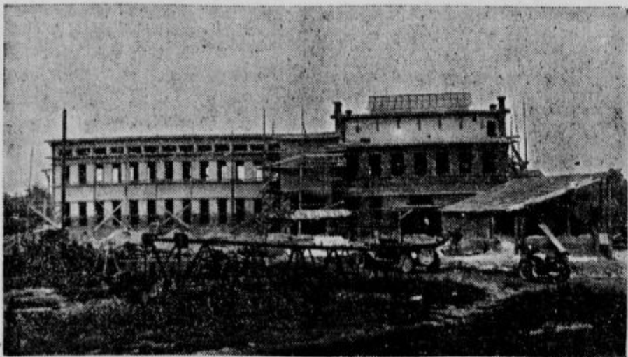
Glavna transformatorska postaja Kranjskih deželnih elektraren na Črnučah. V tej postaji se bo transformirala visoka napetost 60.000 voltov, ki bo prihajala iz Velenja, v nižjo napetost, katero bodo dalinovodi odvajali v lokalne transformatorske postaje v posameznih krajih.
