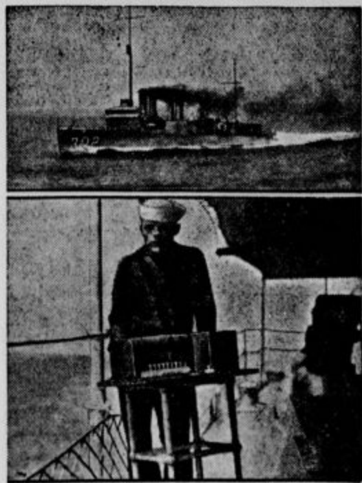
Ameriški manevri s ladjami, ki jih krmarijo iz dalje s pomočjo radia. Zgoraj ladja brez posadke, spodaj radioaparati, s katerim iz dalje vodijo ladjo. Topove na ladji prožijo z ladje spremljevalke — istotako iz dalje.
