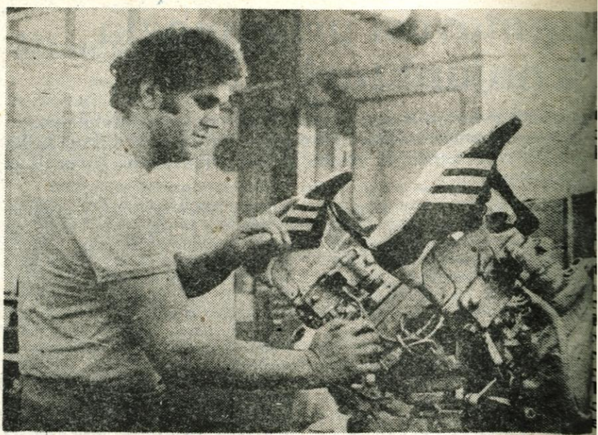
Z najnovejšimi stroji za direktno brizganje podplatov na zgornje dele povečalo število dnevno izdelane športne obutve na 7500, sčasoma pa naj tudi na številko 10.000 do 12.000 parov dnevno. — Foto: F. Perdan
