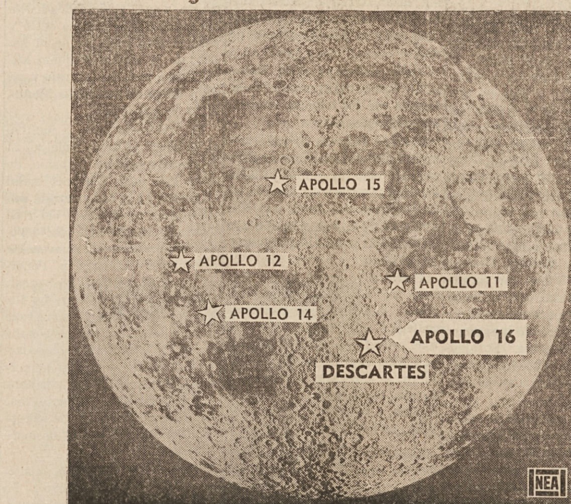
APOLLO 16 BO PRISTAL NA PLANOTI DESCARTES — Slika kaže kraje pristankov dosedanjih in nove odprave na Luno. Planota Descartes, kjer bo pristal Apollo 16, je pokrita z vulkani, med katerimi sodijo, da bi bilo mogoče najti prvotne dele Lunine skorje.
