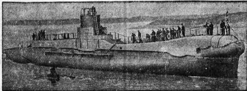
Angleška podmornica »Triton«, o kateri je britanska admiraliteta z obžalovanjem sporočila, da jo je treba smatrati za izgubljeno. V morje so jo spustili leta 1937. Imela je šest cevi za spuščanje torpedov.
