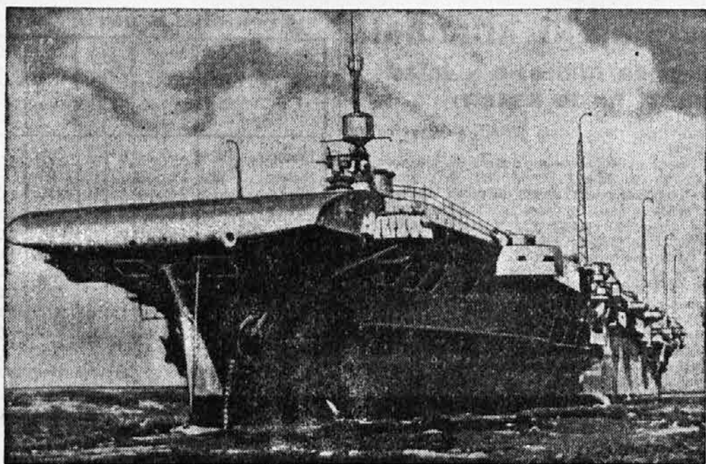
»Illustrious«, slovita angleška 23.000 tonska ladja-letališče, o kateri so zadnjič, ko se je udeležila bitke v Sicilskem prelivu, poročali, da je bila hudo poškodovana, včeraj pa je londonski radio povedal, da je sama priplula v Aleksandrijo. Na njej je prostora za 72 letal.
