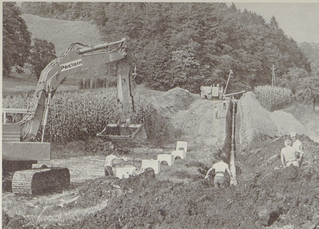
Polaganje plinovoda med Trojanami in Lukovico (Črni graben)
