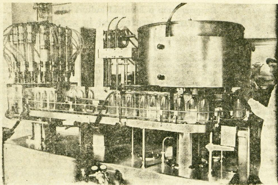
Polnjenje olja v plastične steklenice je povsem avtomatizirano. Pri kontroliranju so potrebni le štirje delavci — Foto: F. Perdan
