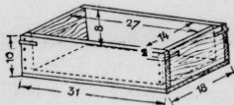
Naprava zidakov (slika 2.)
