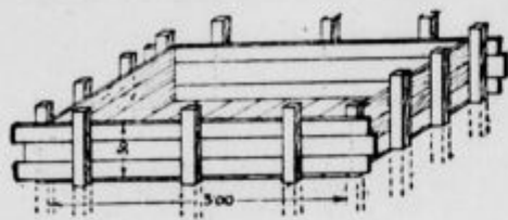
Obdelava ilovice (slika 1.)
