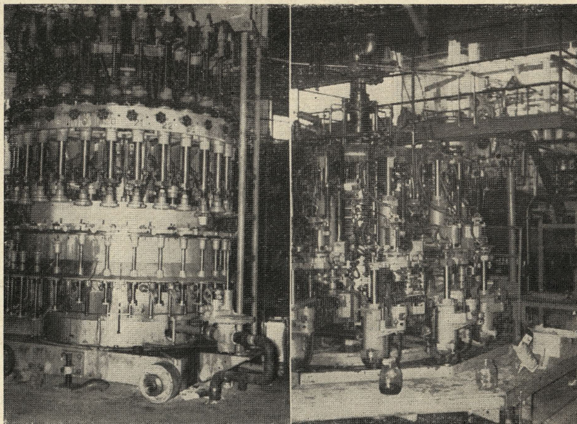
Stroja za izdelavo kozarcev na sliki: desni stroj HARDFORT že obratuje; levi ELDRET, ki je namenjen obžiganju kozarcev pa bo začel obratovati v teh dneh.
