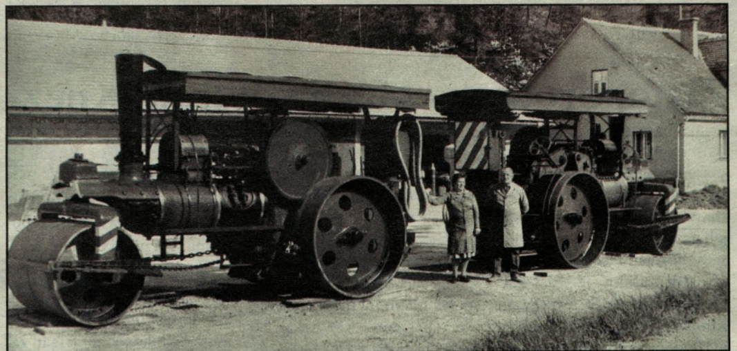
Znani zbiralec in ljubitelj parnih strojev Anton Cizej iz Griž je sredi meseca ponovno spravil v pogon svoj parni valjar iz leta 1935. Navdušeni so bili predstavniki železniškega muzeja z direktorjem Mladenom Bogičem in urednik angleške revije Old Glory Derek Rayner, ki bo našega rojaka predstavil v svoji reviji.
