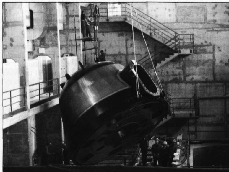
Montaža opreme v strojničnem delu HE Boštanj
